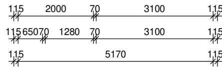
eerste verdieping
