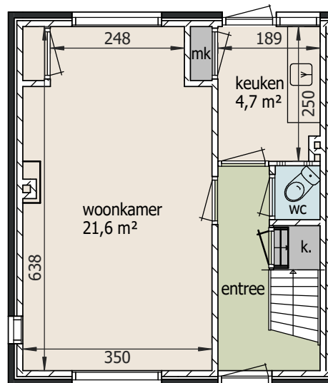
begane grond
