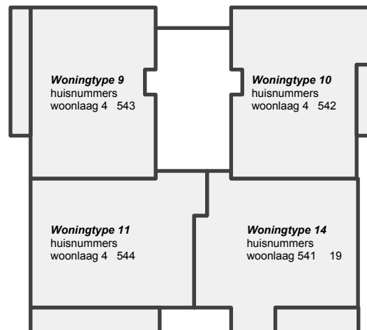
GEBOUW C woonlaag 4
