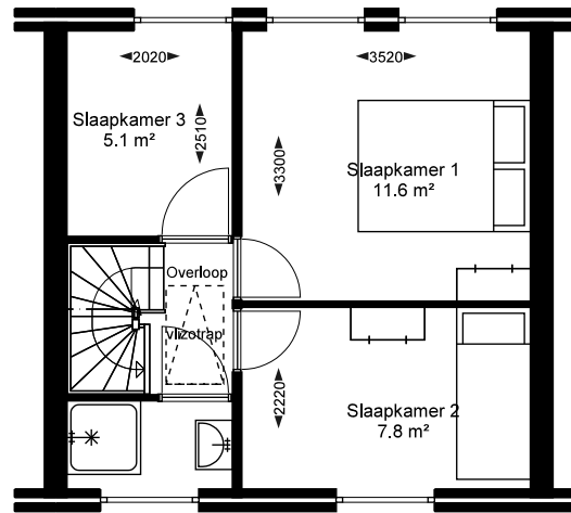
1e verd
