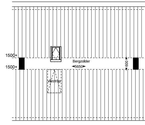
2e verd
