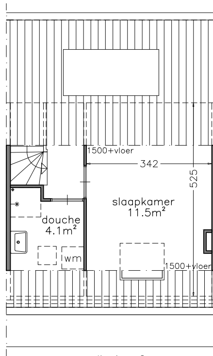
verdieping 2
