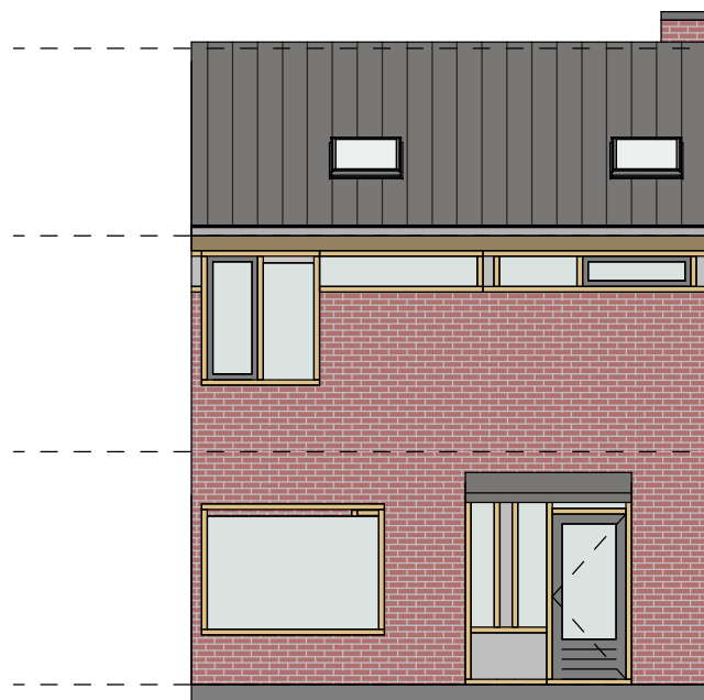
voorgevel
