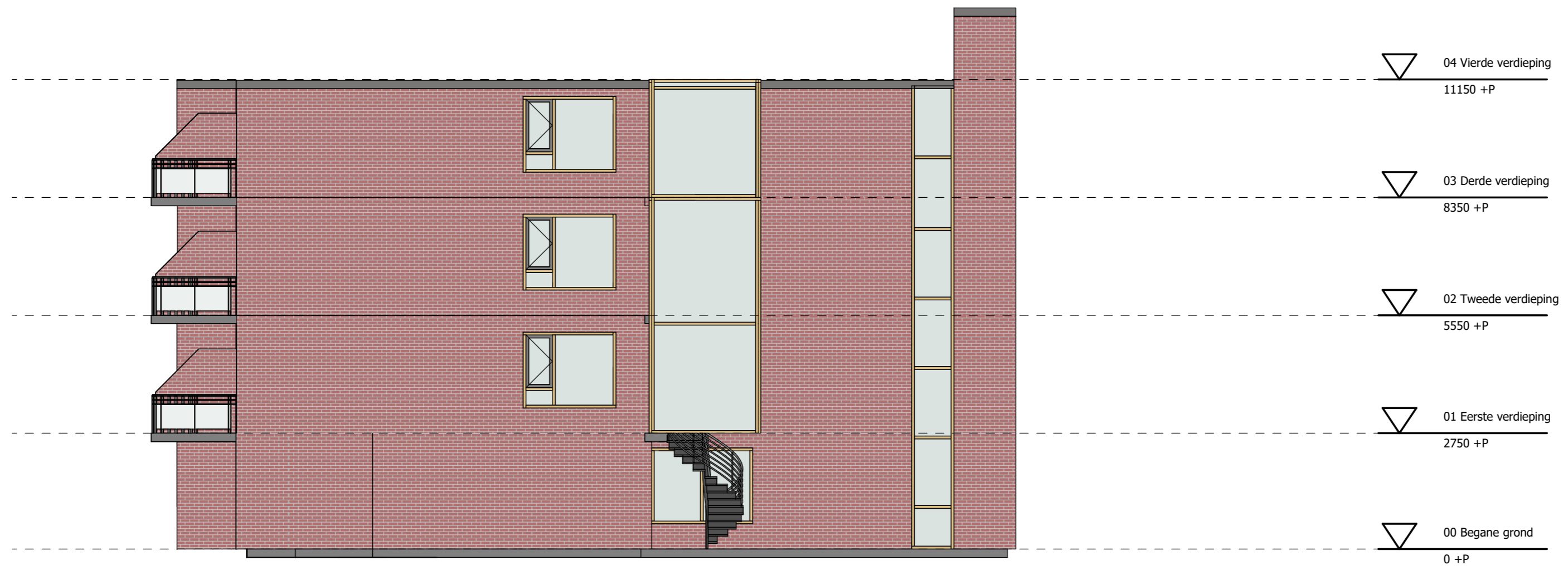
linkergevel
