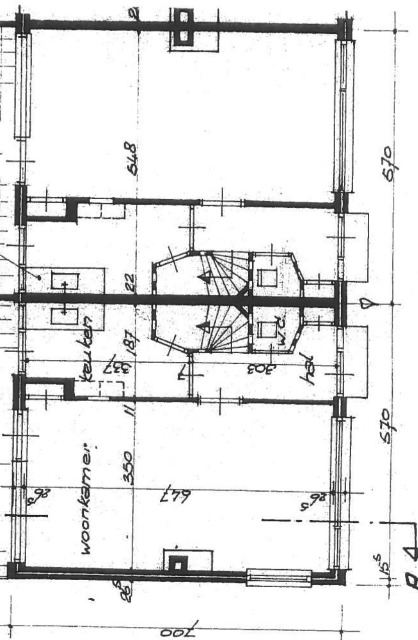
begane grond
